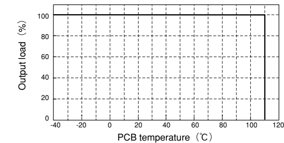
図1-12 PAE100S48基板温度による出力ディレーティング
