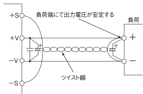
図9-1 リモートセンシングする場合
