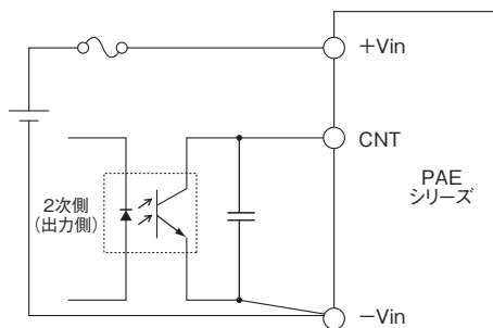
図10-1 接続例
