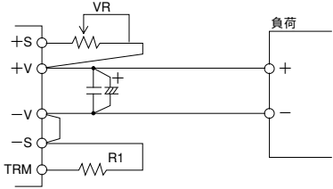
図2-5 外付け抵抗の接続例
