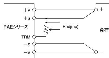
図2-3 可変抵抗接続(2)
