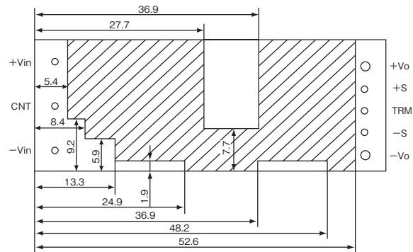
図2-1 パターン配線禁止領域
