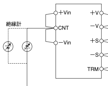
図20-1 絶縁抵抗試験方法
