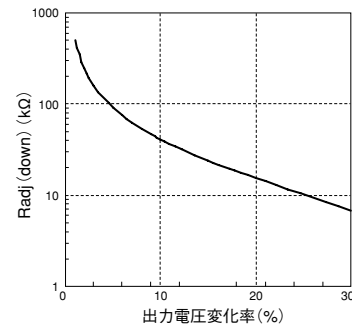
図2-2 △(%)對外付け抵抗(1)
