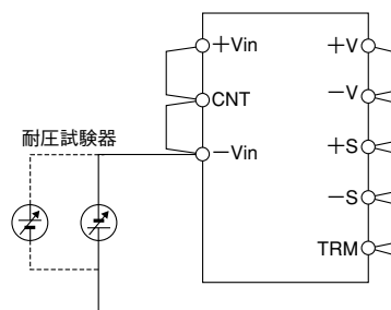
図19-1 入力ー出力間耐電圧試験方法
