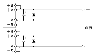
図12-1 出力電圧積み重ね直列運転
