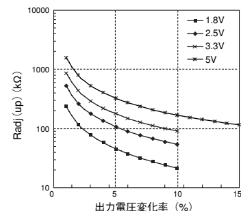
図2-4 △(%)對外付け抵抗(2)
