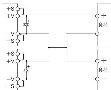
図12-2 正負出力使用の直列運転
