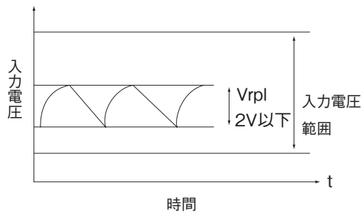
図1-1 入力リップル電圧
