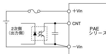
図10-1 接続例
