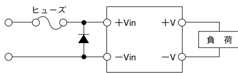
図1-5 入力の逆接続保護
