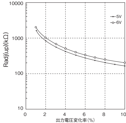
図2-4 \Delta(\%) 對外付け抵抗(2)
